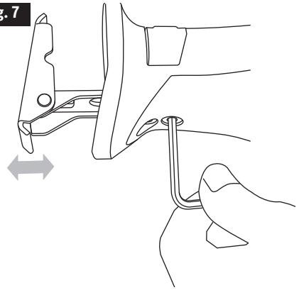
Placa-Base Ajustable
