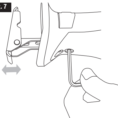
Sabot Réglable
